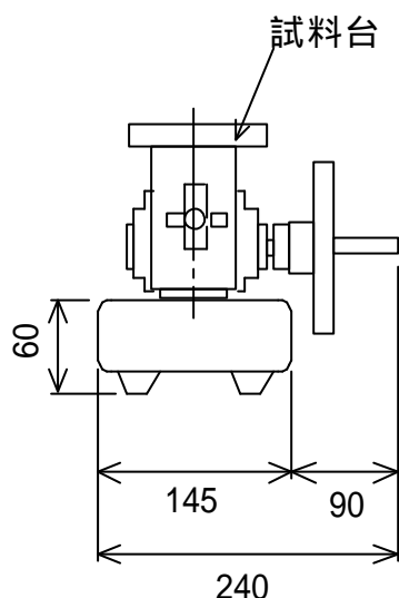
外觀寸法図
